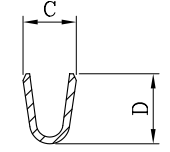
SEC.B-B'
